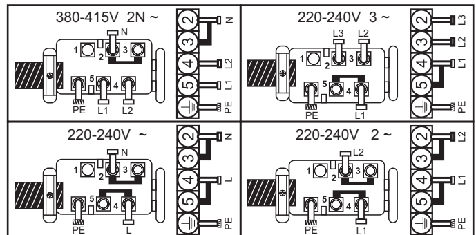
L1 / L2 / L3 = Фаза N = Нуль PE = Заземлення
