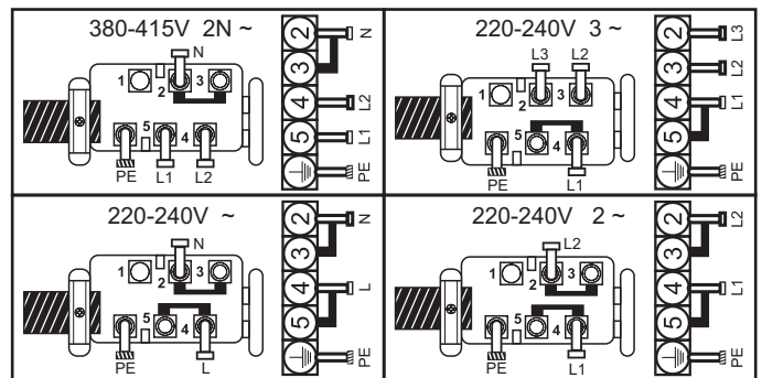
L1 / L2 / L3 = Phase N = Neutre PE = Terre
